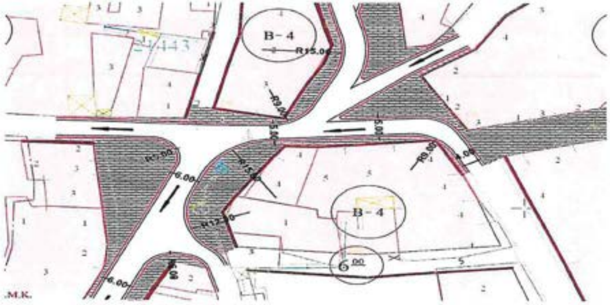
Şekil-3 Geçici Kavşak Düzenlemesi Vaziyet Planı
